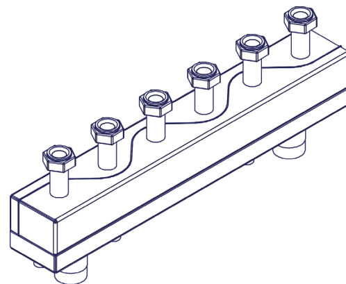
Vedere isometrică
