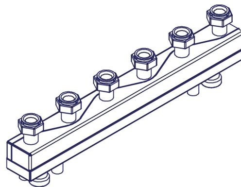
Vedere isometrică
