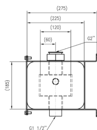
Vedere laterală
