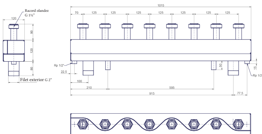
Vedere laterală
