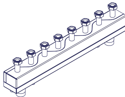
Vedere isometrică
