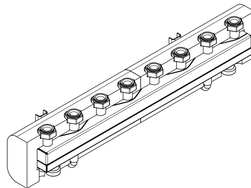
Vedere isometrică
