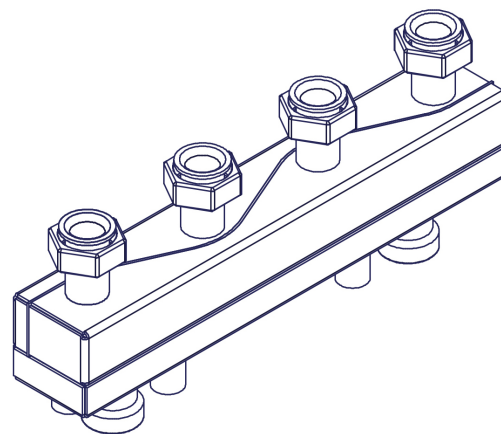
Vedere isometrică
