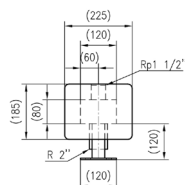
Vedere laterală
