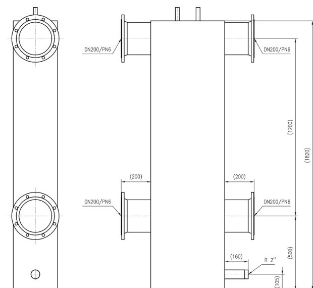
Vedere laterală
