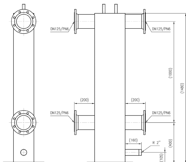
Vedere laterală
