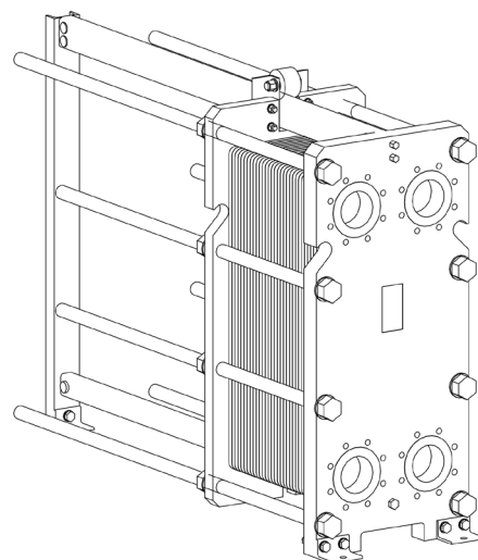
vedere isometrică RLG-21-150
