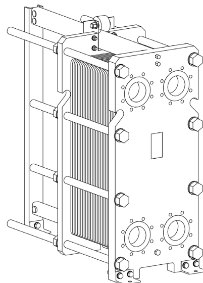
vedere isometrică RLG-21-140
