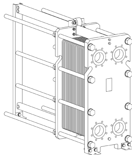
vedere isometrică RMG-21-170
