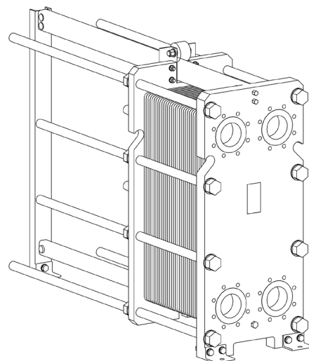
vedere isometrică RHG-21-180
