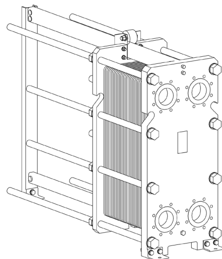
vedere isometrică RHG-21-170
