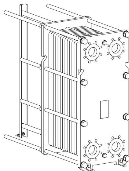
vedere isometrică RLG-19-160
