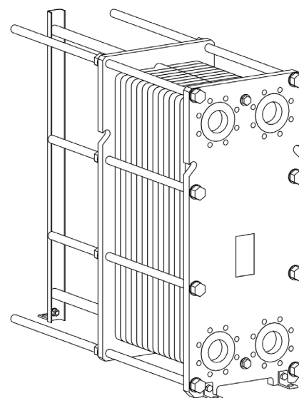
vedere isometrică RLG-19-150
