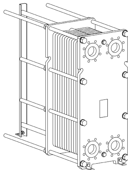
vedere isometrică RLG-19-130
