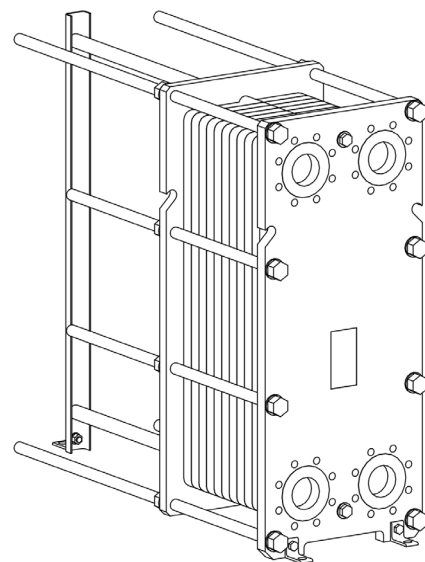
vedere isometrică RLG-19-120
