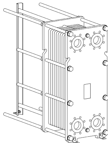
vedere isometrică RLG-19-110
