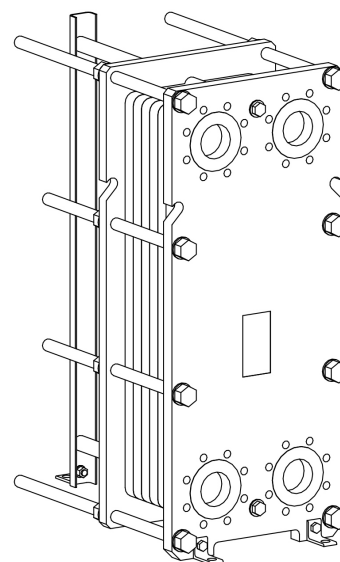
vedere isometrică RLG-19-70
