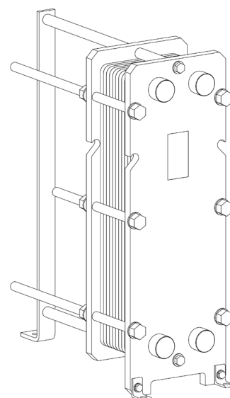
vedere isometrică RLG-14-55
