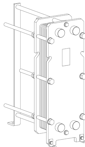
vedere isometrică RLG-14-45
