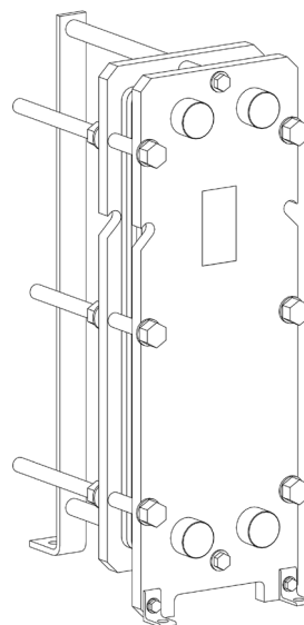
vedere isometrică RLG-14-25
