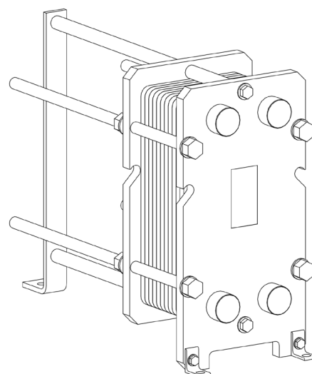
vedere isometrică RMG-07-60
