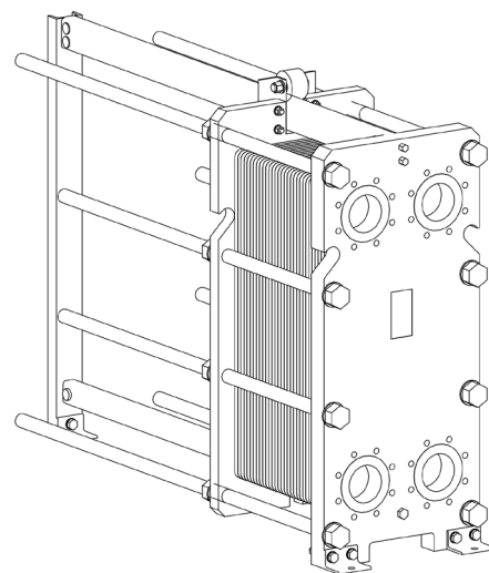
vedere isometrică RMG-21-150
