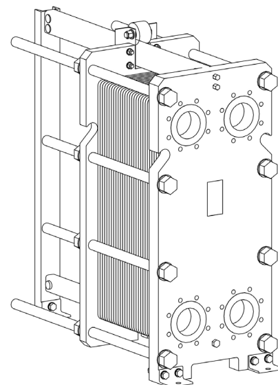
vedere isometrică RMG-21-140
