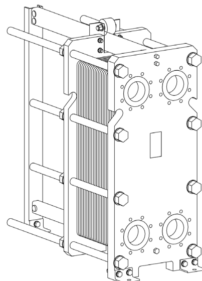
vedere isometrică RMG-21-120
