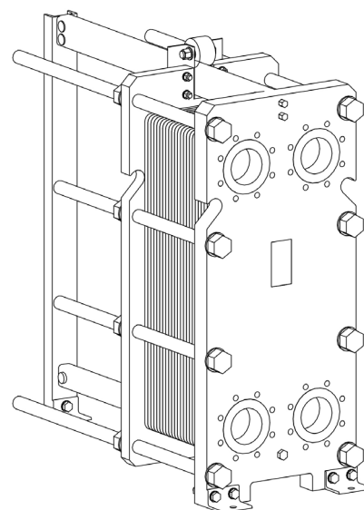
vedere isometrică RMG-21-110
