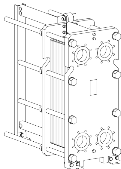
vedere isometrică RMG-21-100
