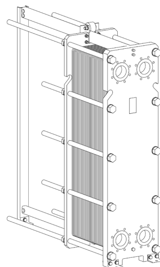
vedere isometrică RHG-51-180
