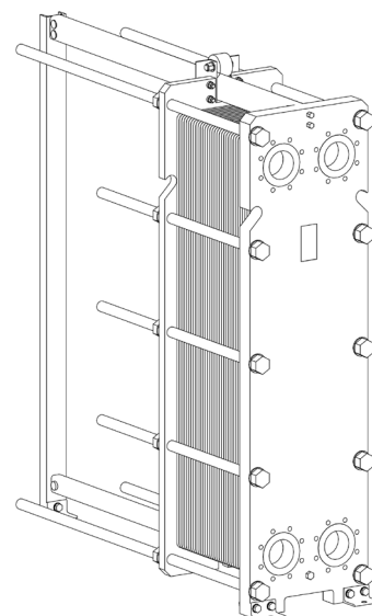
vedere isometrică RHG-51-160
