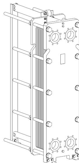
vedere isometrică RHG-51-85
