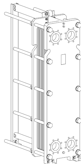
vedere isometrică RHG-51-75
