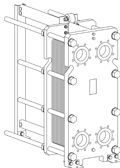
vedere isometrică RHG-21-90
