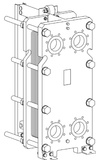
vedere isometrică RHG-21-60
