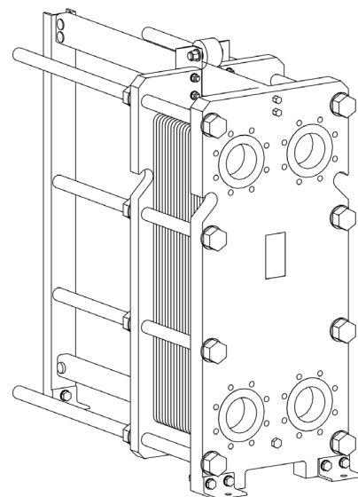
vedere isometrică RMG-21-90
