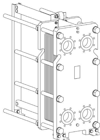
vedere isometrică RMG-21-80
