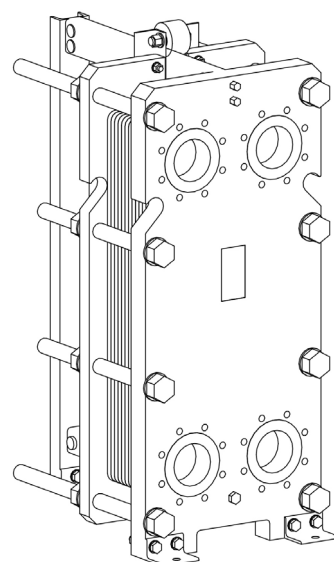
vedere isometrică RMG-21-60
