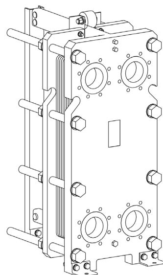
vedere isometrică RMG-21-50
