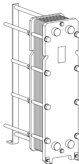
vedere isometrică RHG-20-55
