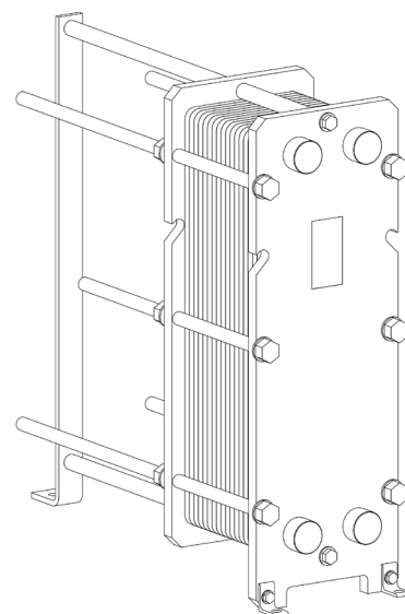
vedere isometrică RHG-14-85
