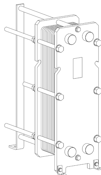
vedere isometrică RHG-14-65
