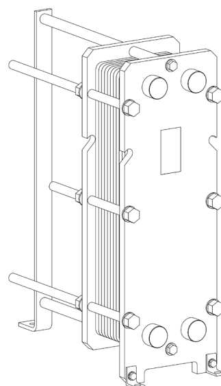
vedere isometrică RHG-14-55
