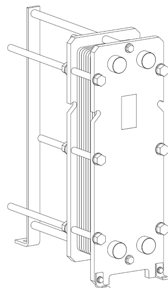
vedere isometrică RHG-14-45
