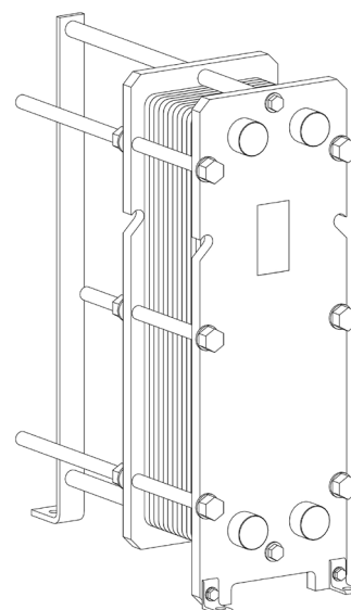
vedere isometrică RMG-14-65
