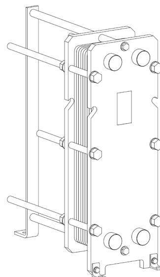
vedere isometrică RMG-14-45
