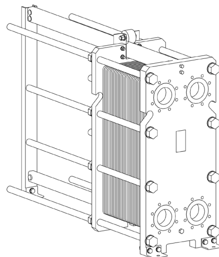
vedere isometrică RHG-21-160
