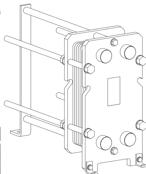
vedere isometrică RHG-07-40
