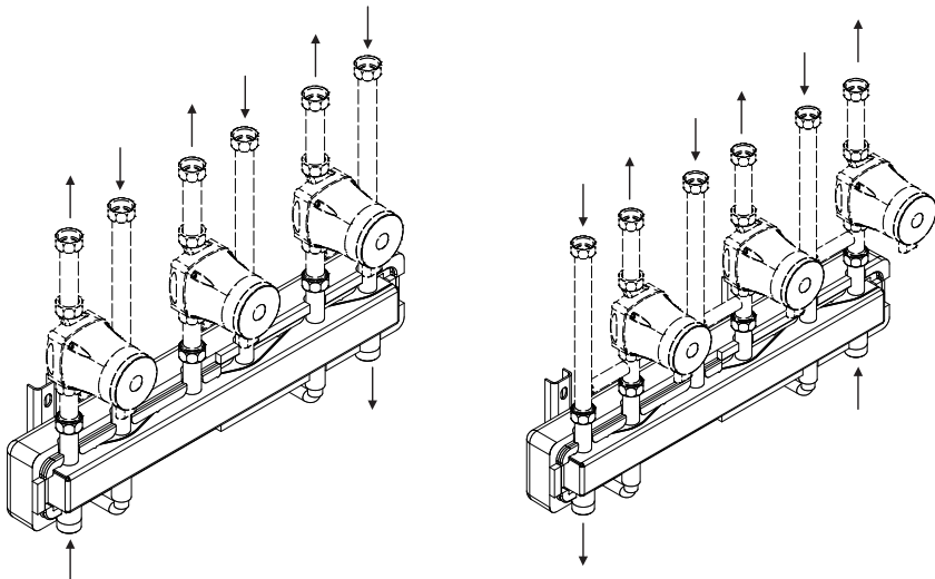
Für 3 / 5 / 7 ... Heizkreise / Pentru 3 / 5 / 7 ... circuite de încălzire
