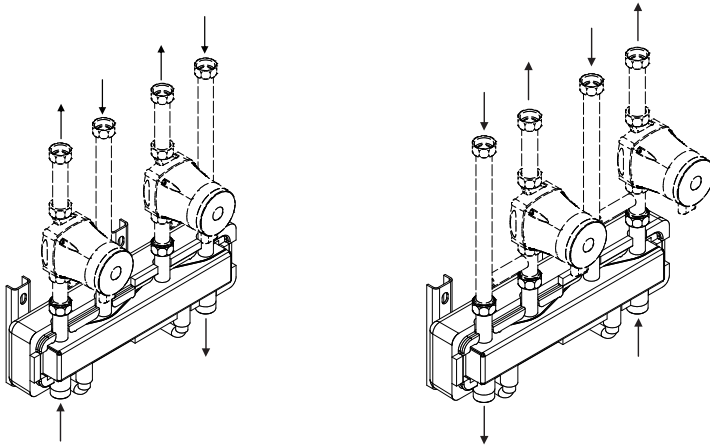
Für 2 / 4 / 6 ... Heizkreise / Pentru 2 / 4 / 6 ... circuite de încălzire
